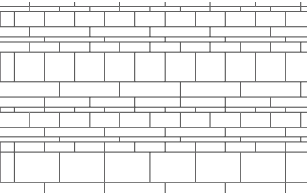
Lauferverband, gemixt, Formate: S2/-3/-4, M2/-3/-4, L2/-3/-4, XL2/-3/-4
