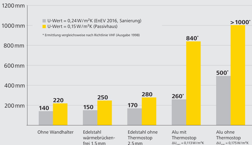
Erforderliche Dämmstoffdicken unter Berücksichtigung von Wärmebrücken durch metallische Unterkonstruktion für bestimmte U-Werte.
